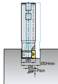
3. Zirkularfräsen einer Durchgangsbohrung
